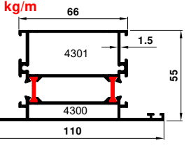
55-1720-1721 2.977 kg/m
