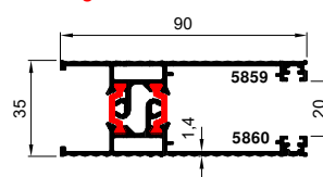
5859-5860 1.651 kg/m
