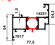
70-7017-14251 1.616 kg/m
