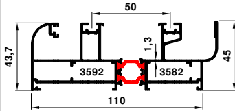
3592-3582 2.140 kg/m
