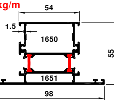
55-4300-4302 2.151 kg/m
