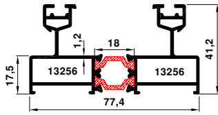
3592-3582 2.140 kg/m
