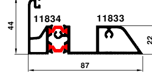
13008 0.205 kg/m
