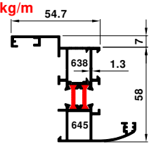
50-13159-13160 1.497 kg/m
