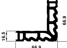
11627 2.929 kg/m
