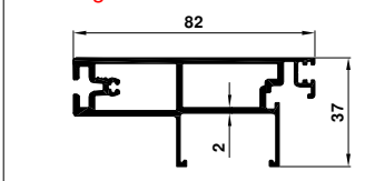
13811 1.456 kg/m
