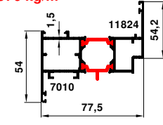
70-7010-11824 1.570 kg/m
