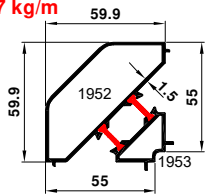
55-1952-1953 1.397 kg/m
