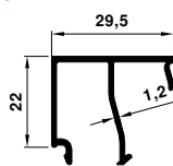
3636 0.321 kg/m
