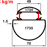
55-1734-1735 1.465 kg/m
