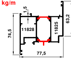
70-7015-11829 2.007 kg/m
