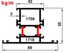
55-4300-4301 2.041 kg/m
