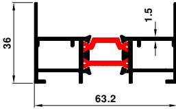
3666-3667 1.357 kg/m
