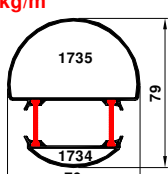
70-1734-1735 1.481 kg/m
