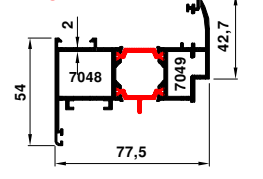
70-7010-14251 1.644 kg/m
