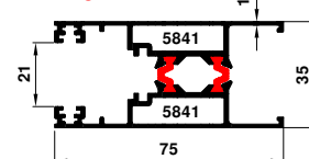
5841-5841 1.400 kg/m
