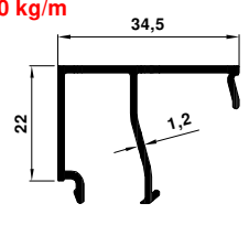
3088 3.498 kg/m
