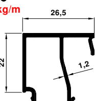
1747 0.340 kg/m
