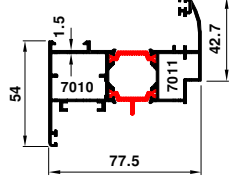
70-7010-7011 1.650 kg/m
