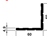
2045 1.436 kg/m
