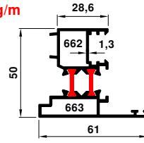
50-662-663 1.177 kg/m
