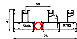
14093-14094 3.436 kg/m
