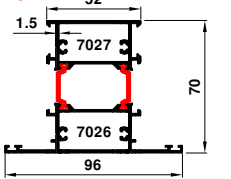
70-7048-7049 1.928 kg/m
