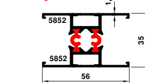
5852-5852 1.066 kg/m
