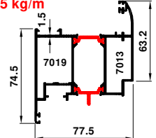
70-7015-14253 1.935 kg/m
