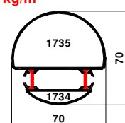
55-1734-1735 1.465 kg/m
