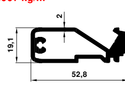
7060 1.007 kg/m
