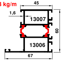
3666-3666 1.306 kg/m
