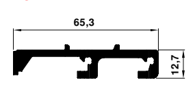
11625 0,990 kg/m
