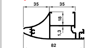
5840 1.030 kg/m
