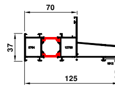
70-7051-7050 2.083 kg/m
