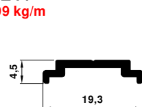
8241 0.099 kg/m
