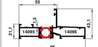
5841-5843 1.749 kg/m
