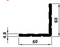
2045 1.436 kg/m
