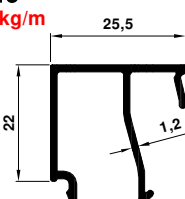
3536 0.329 kg/m
