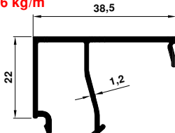
1749 0.356 kg/m
