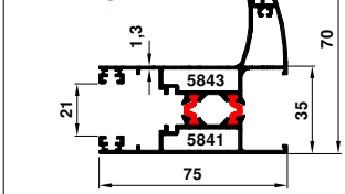
5840 1.030 kg/m
