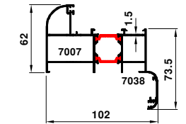
70-7176-7177 2.017 kg/m
