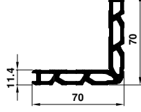
5022 2.245 kg/m
