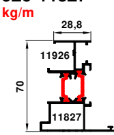
70-11926-11827 1.280 kg/m
