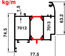
70-11828-7013 2.008 kg/m
