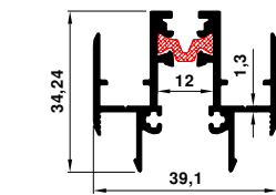
13352-13352 0.715 kg/m
