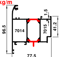
70-12096-7030 2.697 kg/m
