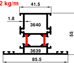
55-5521-5522 2.272 kg/m
