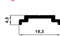
8241 0.099 kg/m
