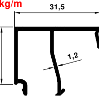
5546 0.271 kg/m
