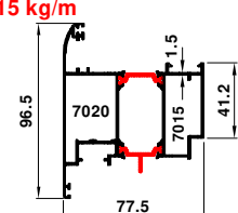
70-7015-11826 1.860 kg/m
