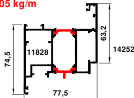
70-7015-7020 2.015 kg/m
