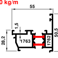
55-1762-1763 1.190 kg/m
