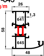
50-13160-13161 1.377 kg/m
