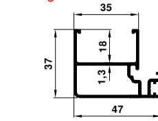
12649 0.666 kg/m
