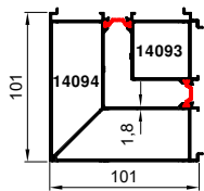
5855-5856 1.535 kg/m
