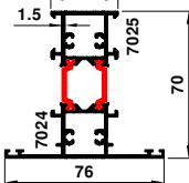
70-7051-11851 1.907 kg/m
