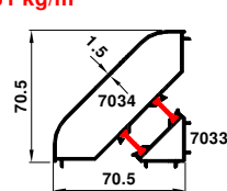
70-11926-11827 1.280 kg/m
