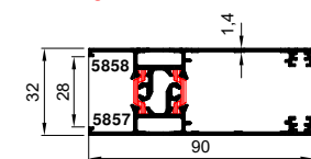
5857-5858 1.629 kg/m
