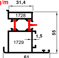
55-1728-1729 1.337 kg/m
