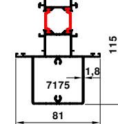
70-7010-11824 1.570 kg/m
