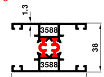
3588-3588 1.134 kg/m
