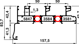
12651-12872 2.203 kg/m
