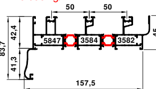
5853-5854 1.315 kg/m
