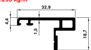
10923 0.295 kg/m
