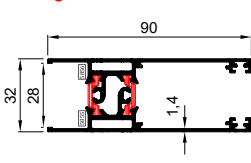
5855-5856 1.535 kg/m
