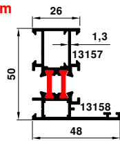
50-638-642 1.232 kg/m
