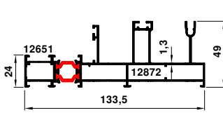
5857-5858 1.629 kg/m
