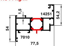
70-7010-14251 1.644 kg/m
