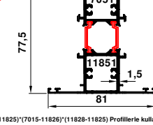
70-8764-7175 2.466 kg/m
