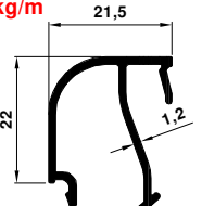
1746 0.279 kg/m
