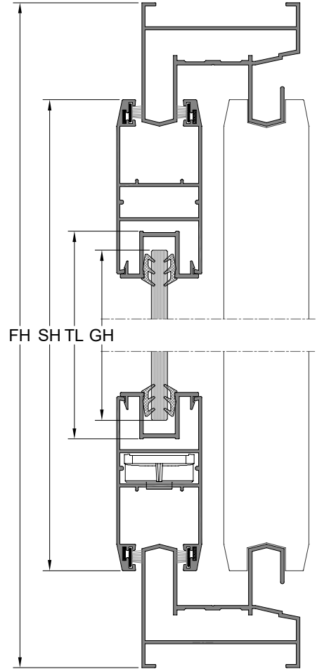
B-B KESİTİ
