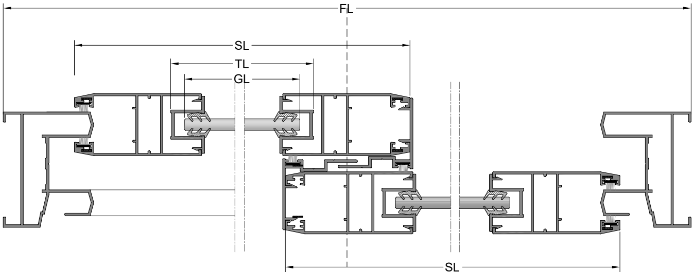
A-A KESİTİ
