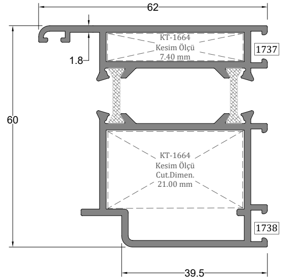
★ Hemiyüz İçe Açılır Kasa Profili SYMMETRICAL INWARD OPENING FRAME PROFILE
