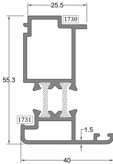
★ Hemiyüz İçe Açılır Adaptör Profili SYMMETRICAL INWARD OPENING FRAME PROFILE
