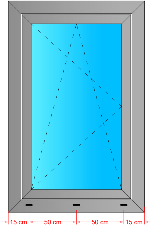
Su Tahliye İşlem Şeması WATER DRAINAGE PROCESS DIAGRAM
