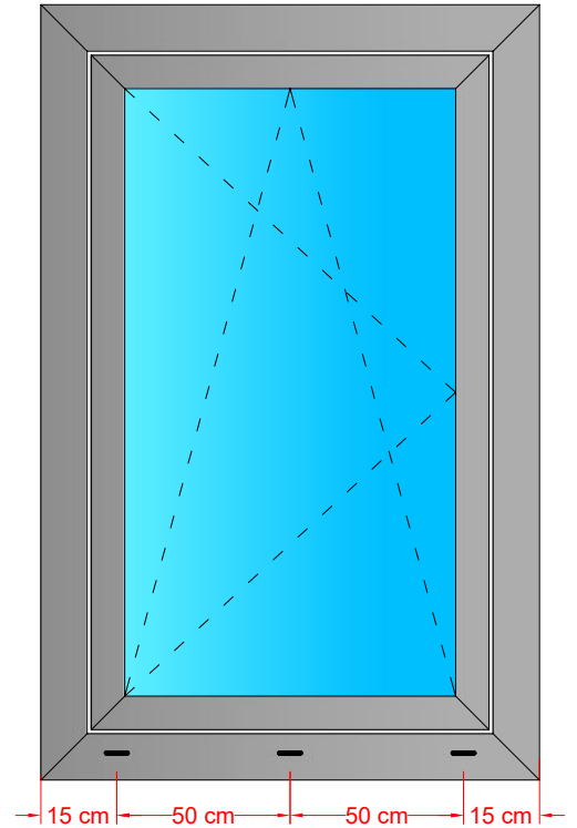
Su Tahliye Delikleri WATER DRAINAGE HOLES
