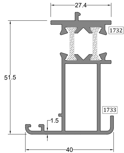
★ Hemiyüz Dışa Açılır Adaptör Profili SYMMETRICAL OUTWARD OPENING FRAME PROFILE
