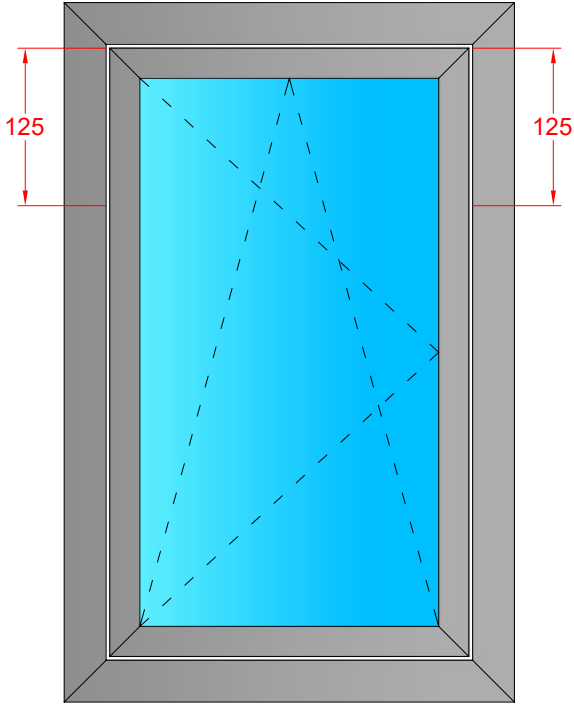
Kanat Üzerinde Basınç Dengeleme DECOMPRESSION IN SASH
