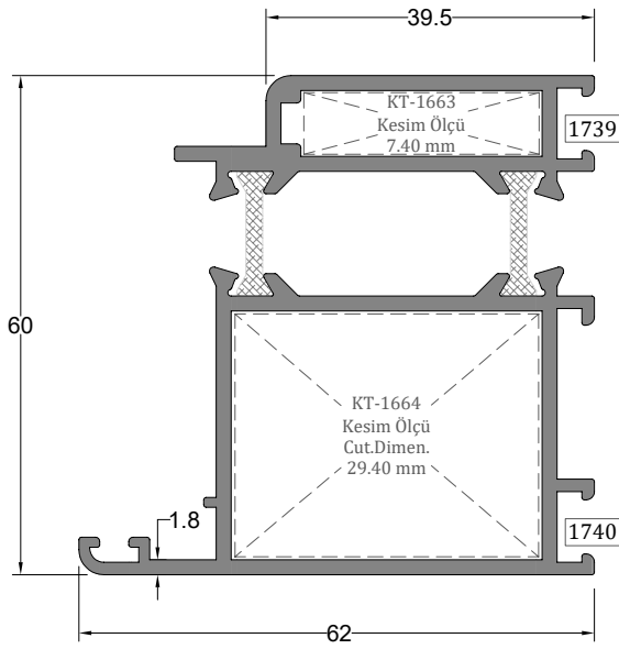
★ Hemiyüz Dışa Açılır Kasa Profili SYMMETRICAL OUTWARD OPENING FRAME PROFILE
